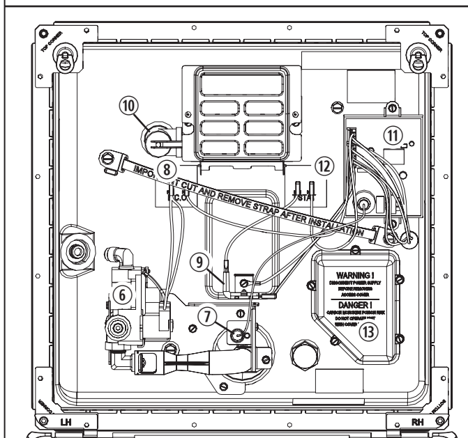
2 WH - 10GEA and WH - 16GEA Emplacements des Composants
