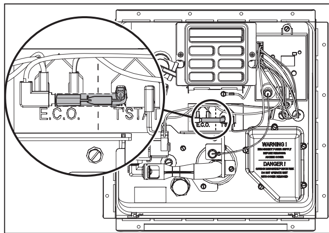
19 Système de coupure thermique
