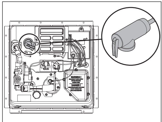
23 Soupape de sécurité P/T
