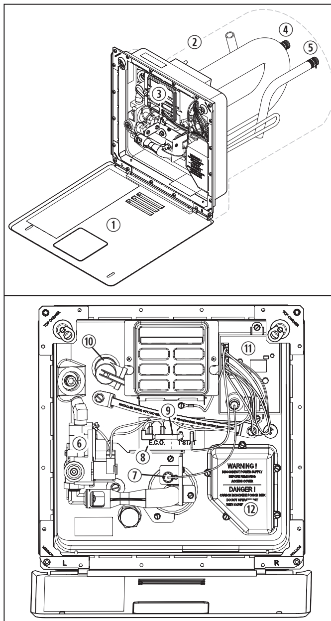
1 WH - 6GA, WH - 6GEA, and WH - 9GEA Emplacements des Composants
