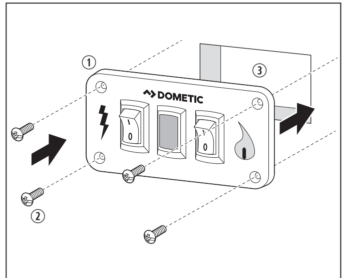
9 Installation de l'interrupteur double
