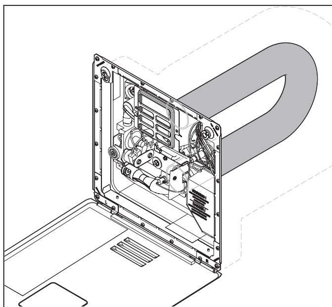
20 Tube du brûleur
