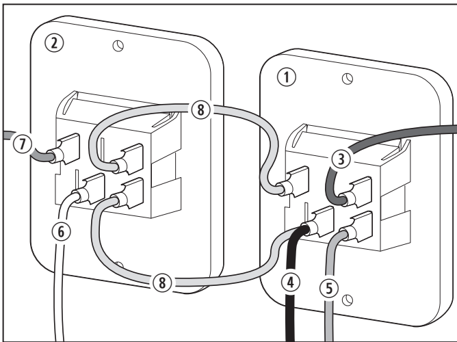
11 Câblage d'un interrupteur simple à fonction combinée
