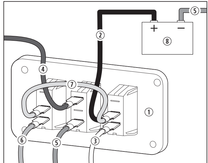
12 Câblage de l'interrupteur double
