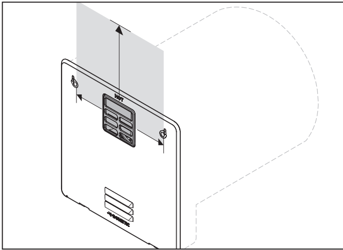
4 Distances minimales de l'évent
