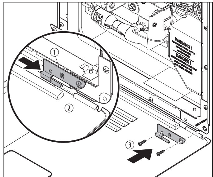
16 Fixation de la charnière droite
