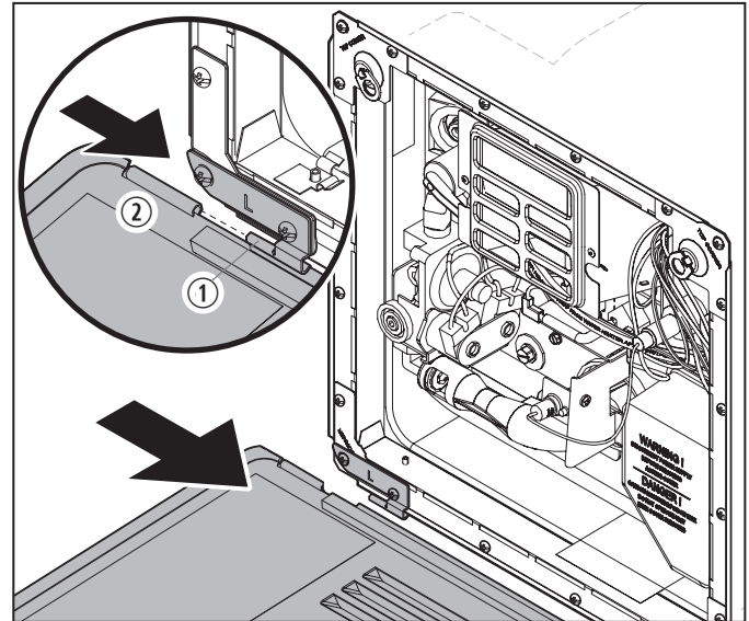
15 Glissement de la trappe d'accès sur la charnière gauche
