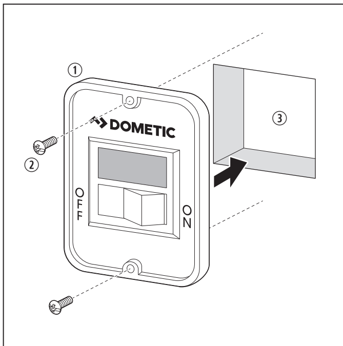
8 Installation de l'interrupteur simple
