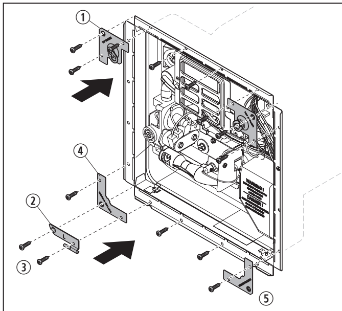
14 Fixer les équerres de fixation et la bride
