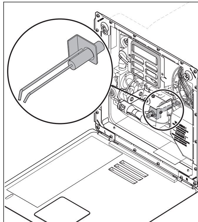
21 Inspection de l'électrode
