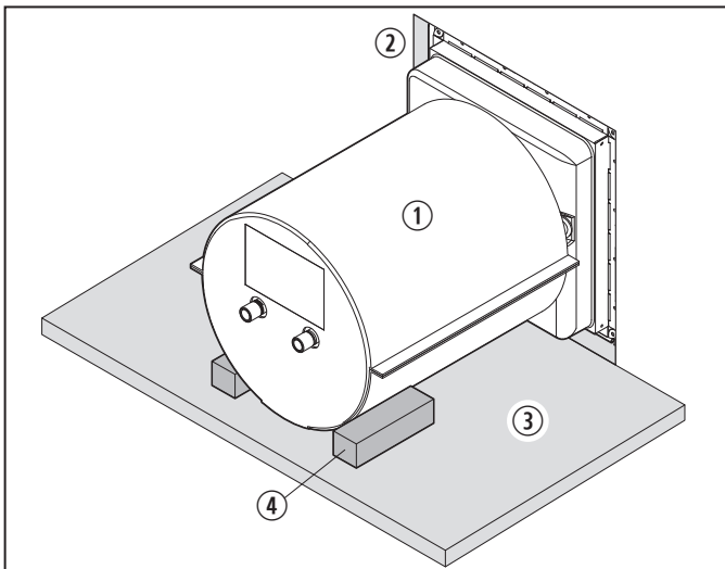
5 Calage du chauffe-eau
