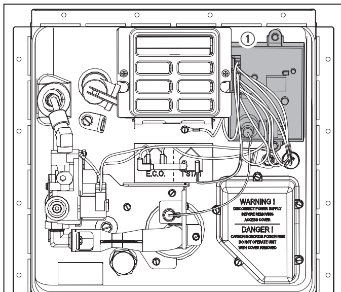
22 Carte contrôleur DSI
