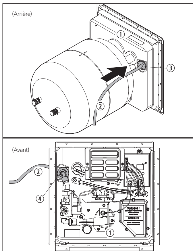
7 Étanchéiser la ligne de gaz avec l'œillet
